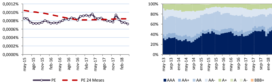
Pérdida Esperada y Clasificación de riesgo de los emisores Fondo Mutuo Solvente BancoEstado
